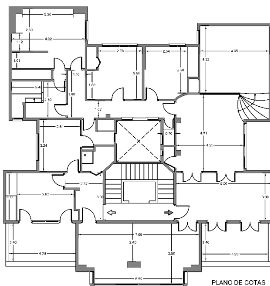
PLANO DE COTAS ESTADO ACTUAL
