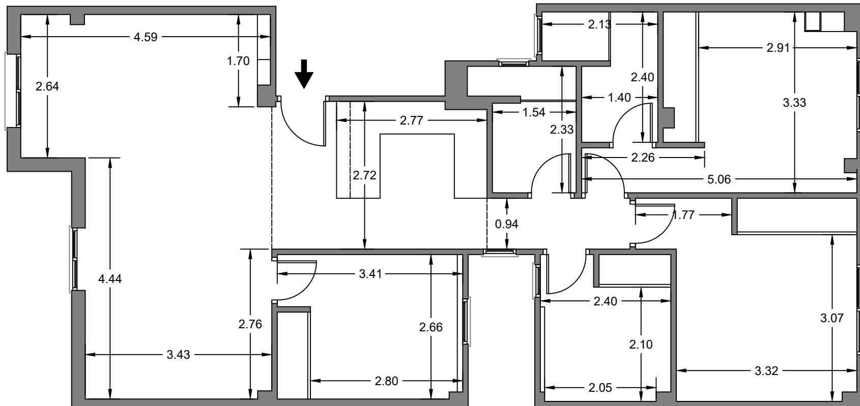
PLANO DE COTAS
